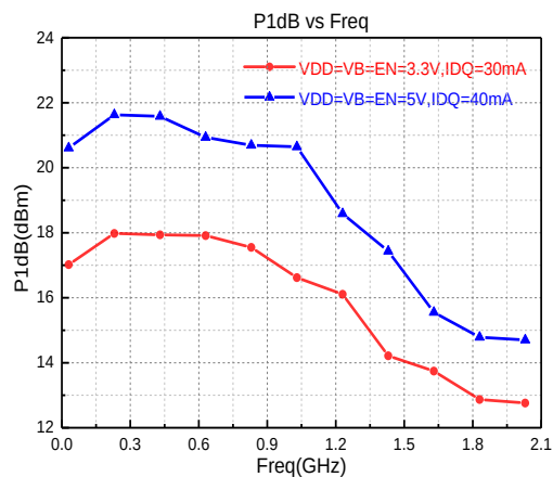
输出 1dB 压缩点曲线
